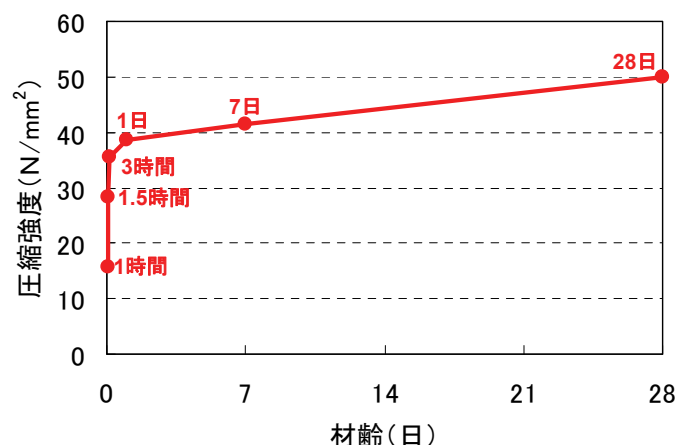
図1 圧縮強度
