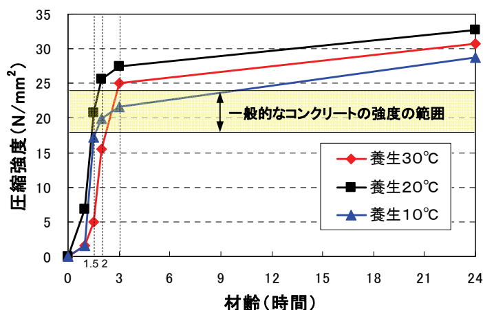
図1 圧縮強度 (φ50mm × h100mm 供試体)
