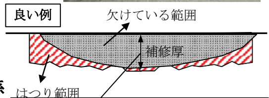
補修箇所の断面図
